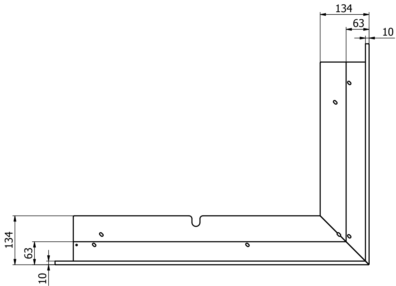
Maskownica 50 płytka
